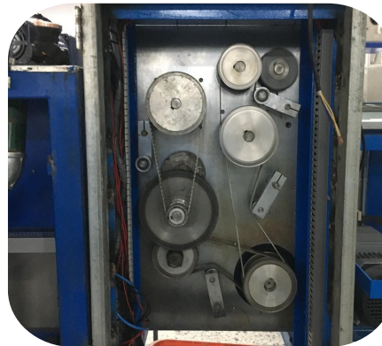
Nâng cấp hệ thống cho máy làm tăm bông tự động
