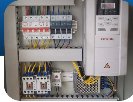
Biến tần GK820 cho Tang Cuốn Cáp
