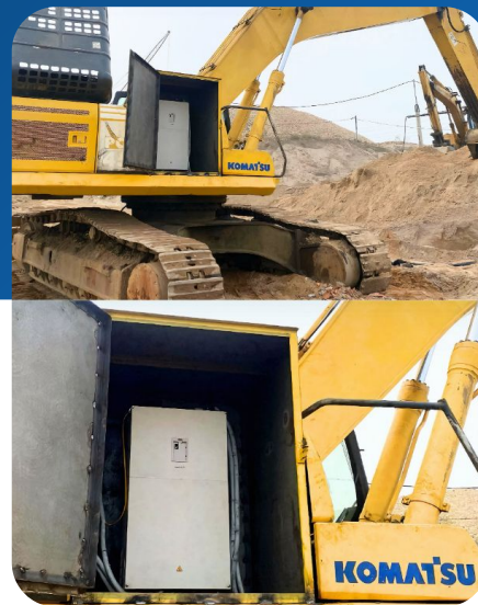
GK620 250Kw cho Máy Xúc Điện
